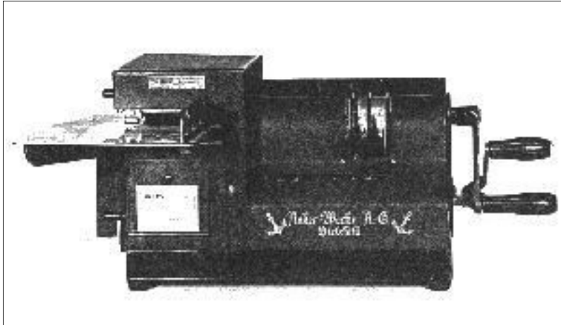
Bild 1 Stempelmaschine
